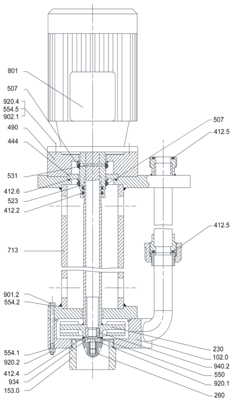
Fig. 3 Unité de pompe avec vis
