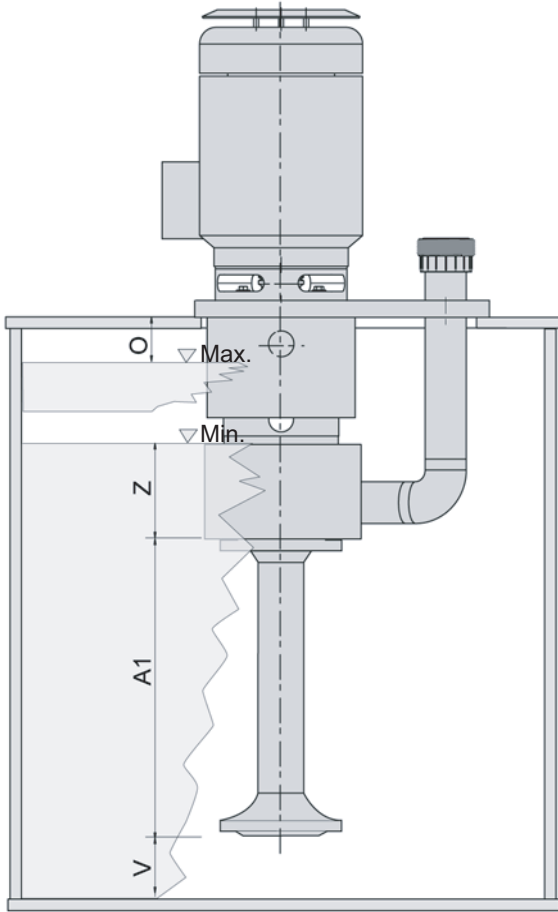
Fig. 5 Hauteurs de remplissage avec extension du tube d'aspiration
