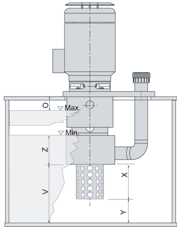
Fig. 6 Hauteurs de remplissage avec crépine
