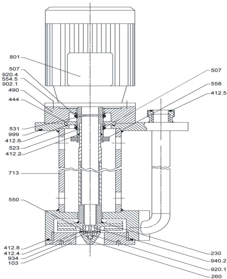
Fig. 4 Unité de pompe sans vis
