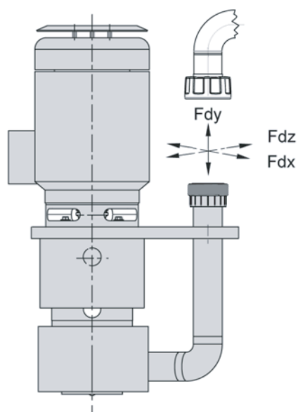
Fig. 7 Forces admissibles à la tubulure de refoulement
